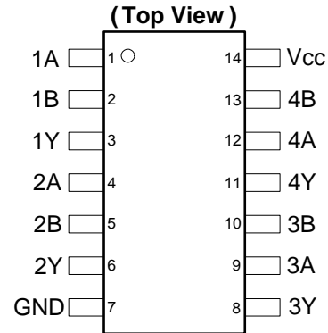
SO-14 / TSSOP-14
